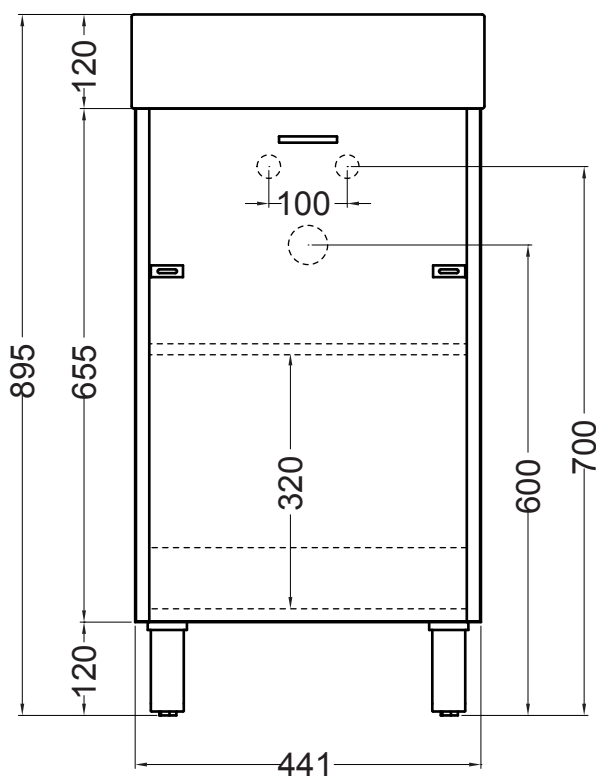
VISTA FRONTALE
