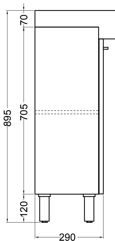
VISTA LATERALE
