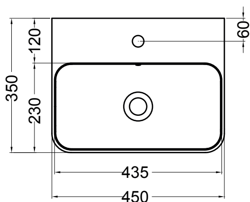
PIANTA
